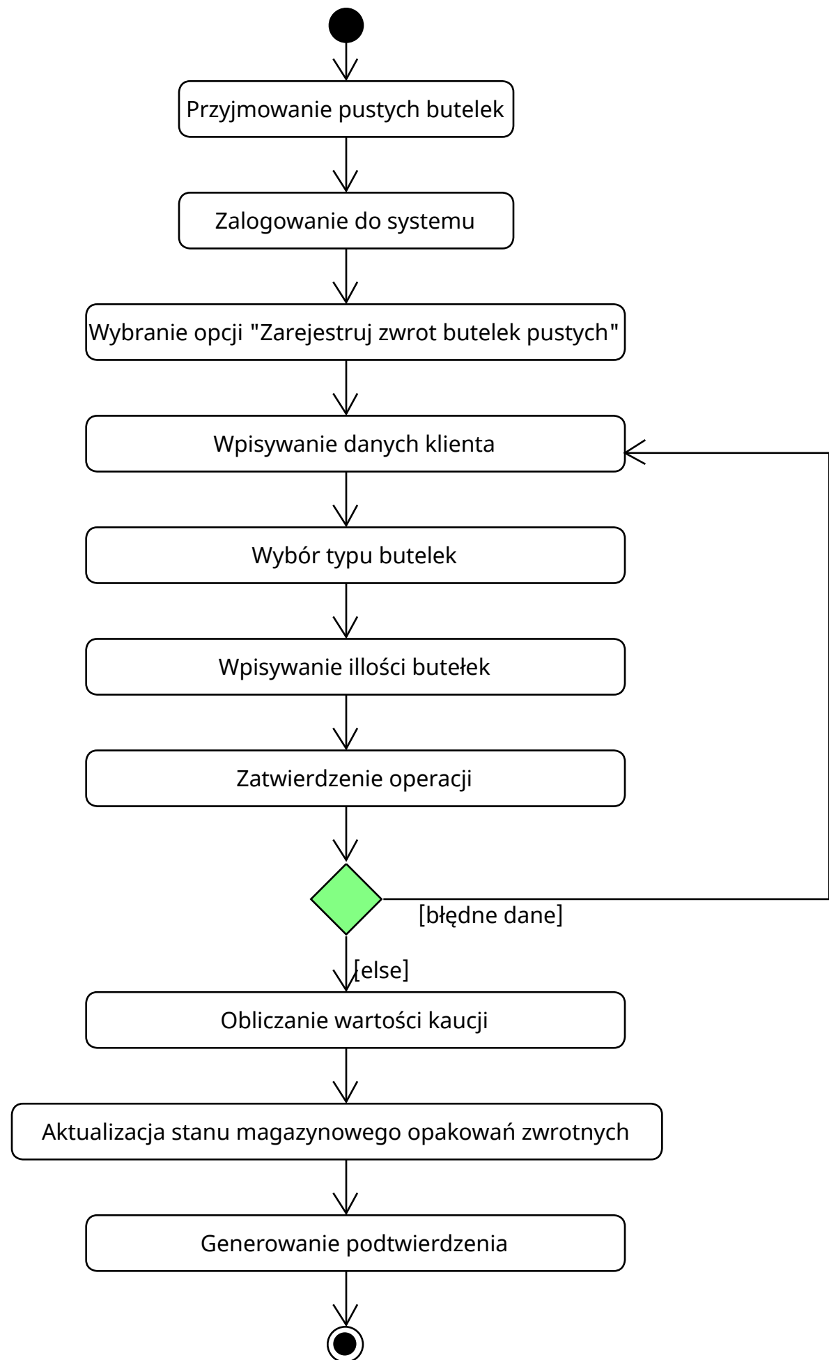
Diagram czynności Przypadek: Zarejestruj zwrot pustych butelek Roman Saienko
